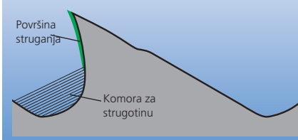
Presjek karoserijske turpije Prikaz konveksnosti
